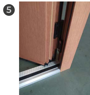
5 ZAPATA INFERIOR Cortavientos con 2 gomas
